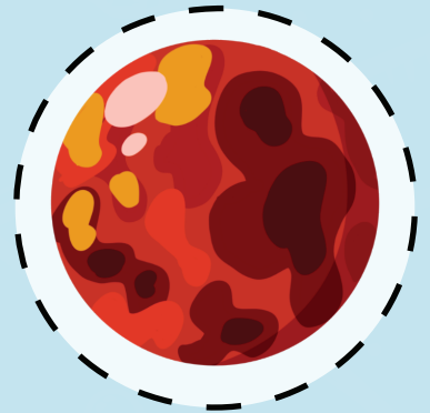
Mars
