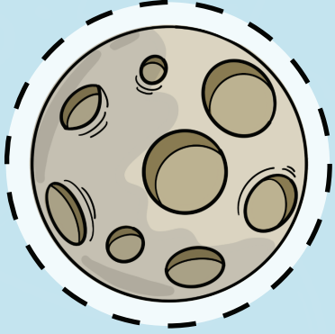
Moon
